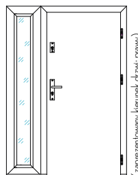
drzwi z dostawką boczną wariant A
